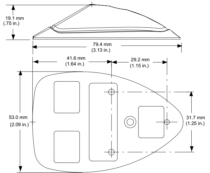
DIMENSIONS • ABMESSUNGEN • DIMENSIONES • DIMENSIONI FIGURE 5 • ABBILDUNG 5 • FIGURA 5
