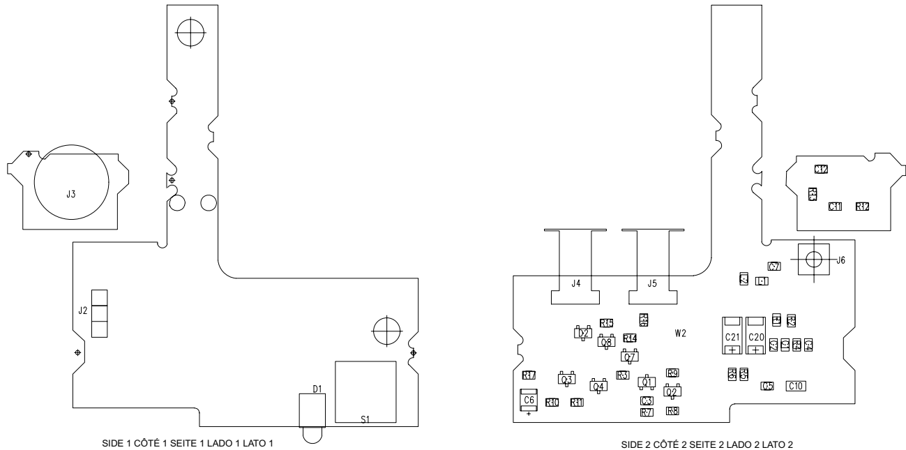
PREAMPLIFIER CIRCUIT BOARD LEGEND • LÉGENDE DU CIRCUIT IMPRIMÉ DU PRÉAMPLIFICATEUR BESCHRIFTUNG DER VORVERSTÄRKER-LEITERPLATTE • LEYENDA DE TARJETA DE CIRCUITOS DE PREAMPLIFICADOR LEGENDA DELLA SCHEDA DI CIRCUITI DEI MODELLI DEL PREAMPLIFICATORE FIGURE 6 • ABBILDUNG 6 • FIGURA 6
