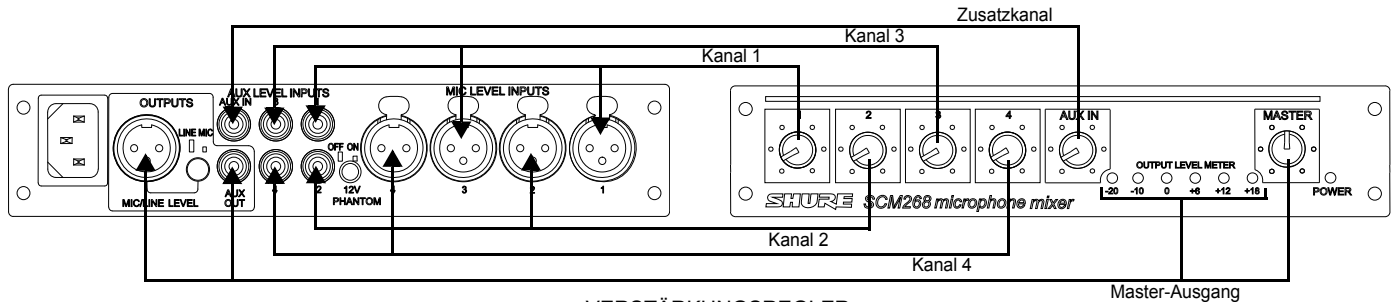
VERSTÄRKUNGSREGLER ABBILDUNG 1
