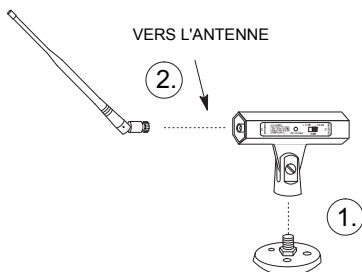
FIXATION DU SUPPORT ET DE L'ANTENNE FIGURE 2
