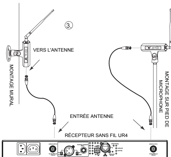
RACCORDEMENT D'UN RÉCEPTEUR FIGURE 3
