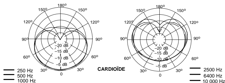
COURBE DE DIRECTIVITÉ TYPIQUE FIGURE 5
