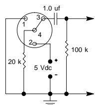
CIRCUIT D'ESSAI FIGURE 1
