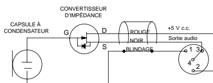
SCHÉMA DE CÂBLAGE DES MICROPHONES SÉRIES WL50/MC50 et WL51/MC51 AVEC CONNECTEUR TA4F FIGURE 6
