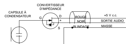
SCHÉMA DE CÂBLAGE DU MICROPHONE SÉRIE WL50X (SANS TERMINAISON) FIGURE 7
