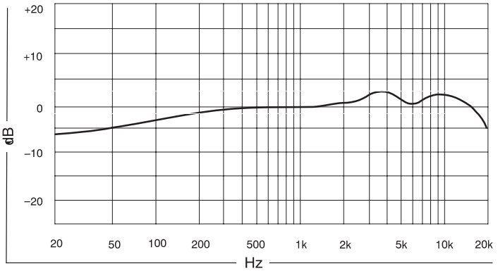
FIGURE 1. RÉPONSE EN FRÉQUENCE TYPIQUE
